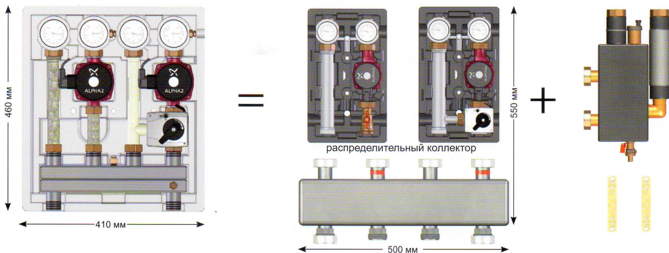
Насосно смесительный модуль Ком- bimix UKMK
